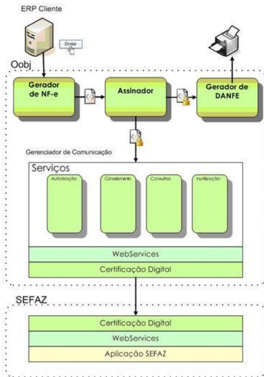
Figura 1 - Arquitetura de Processamento DF-e
